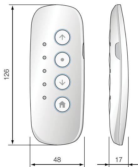
Dimensioni fronte.
